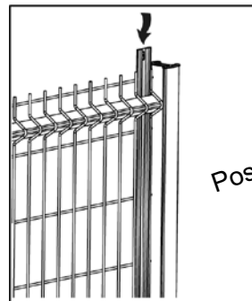
glissez la lame de rive droite
