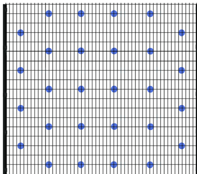
Distribution symétrique du poids avec un remplissage de galets gris ( densité : 1500 \text{ kg/m}^3 ) en combinaison avec système de fixation FASTFIX.
