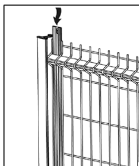
glissez la lame de rive gauche
