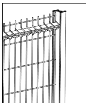
glissez la cornière haute
